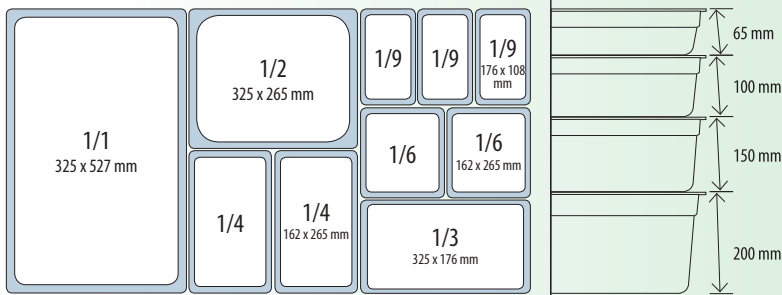
GNP-19100 100 mm 0,75 Lt - 25 Oz 12 pcs /ctn Şeffaf - Siyah Clear - Black 176 x 108 x 100mm
